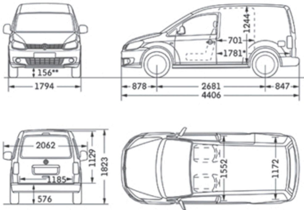
Caddy Panel Van
